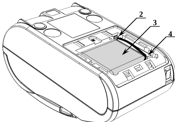
Рисунок 6. Подключение АКБ
